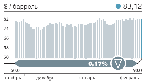
НЕФТЬ BRENT
